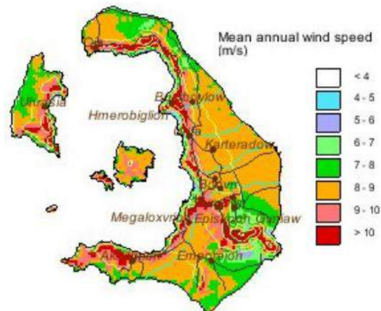
Σχήμα 2.2. Αιολικό δυναμικό
